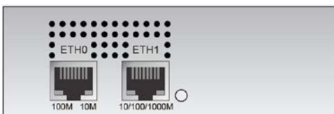
Исполнение /1GE (1 шт 10/100 Мбит/с, 1 шт 10/100/1000 Мбит/с)
